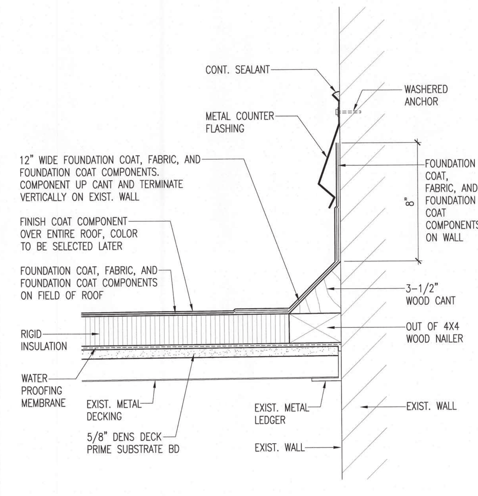
6 WALL FLASHING DETAIL A-3 SCALE: 3"=1'-0"
