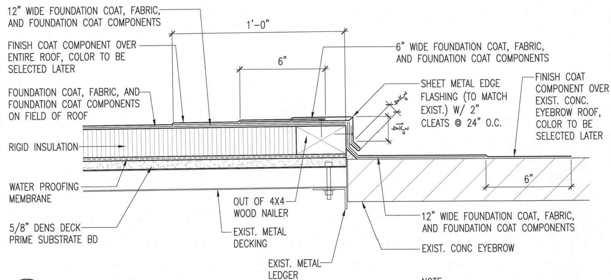
3 ROOF EDGE DETAIL A-3 SCALE: 3"=1'-0"
