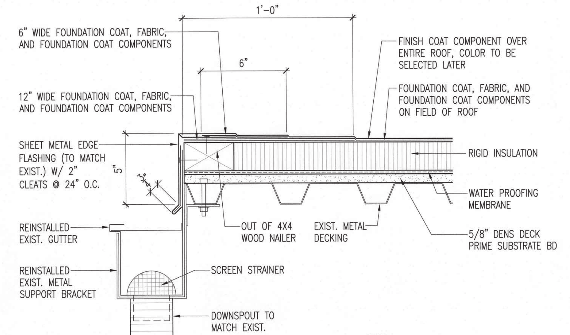
8 ROOF EDGE DETAIL A-3 SCALE: 3"=1'-0"
