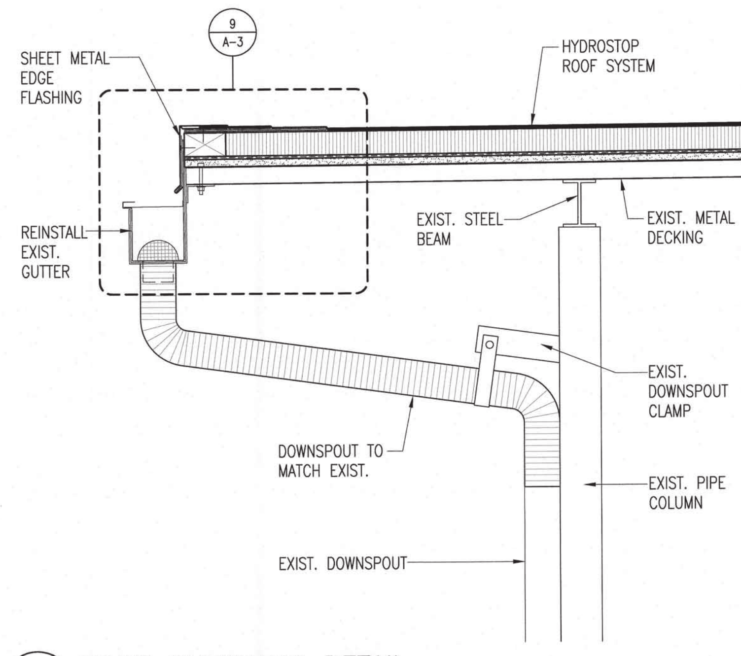
2 ROOF OVERHANG DETAIL A-3 SCALE: 1-1/2"=1'-0"
