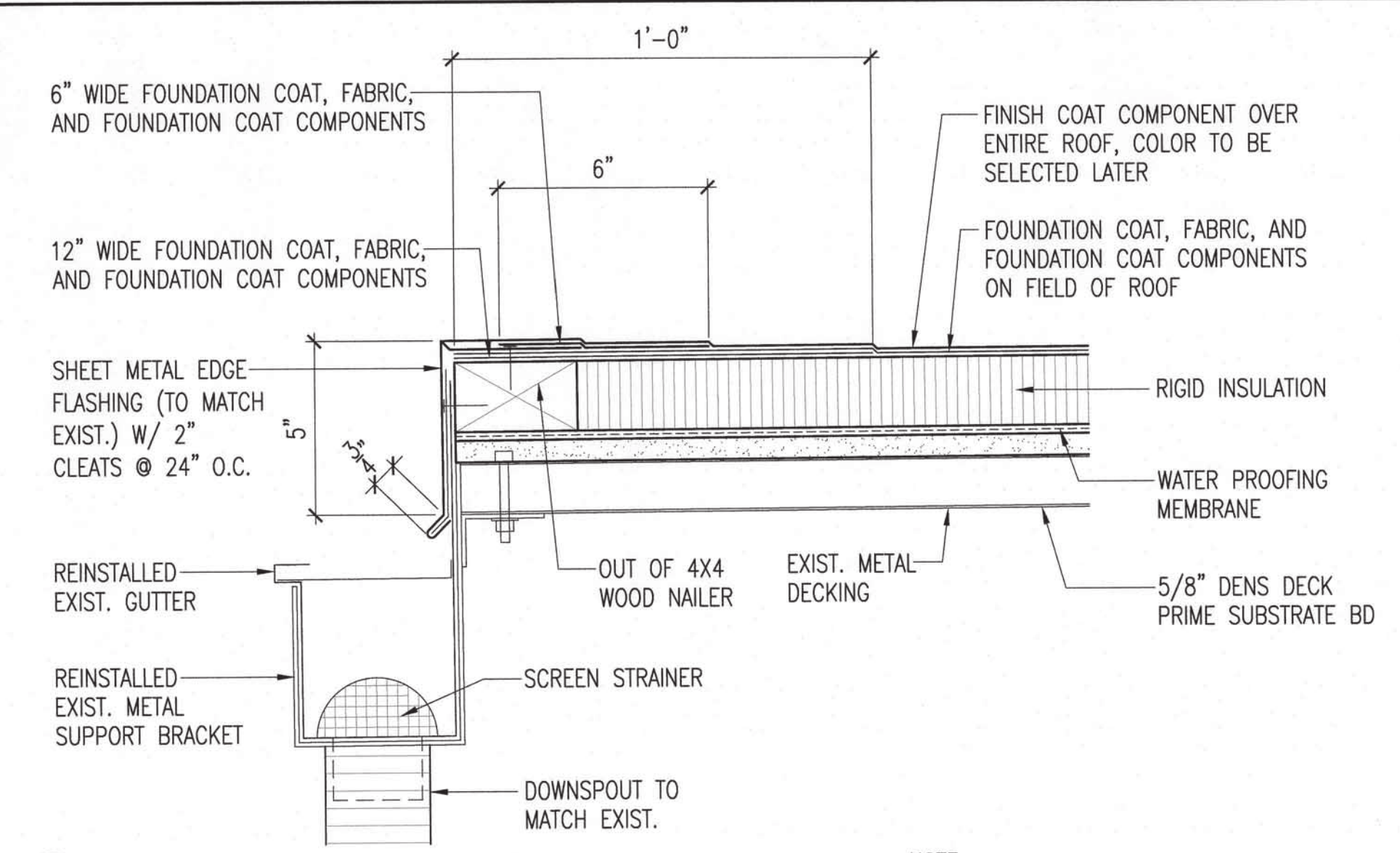
9 ROOF EDGE DETAIL A-3 SCALE: 3"=1'-0"
